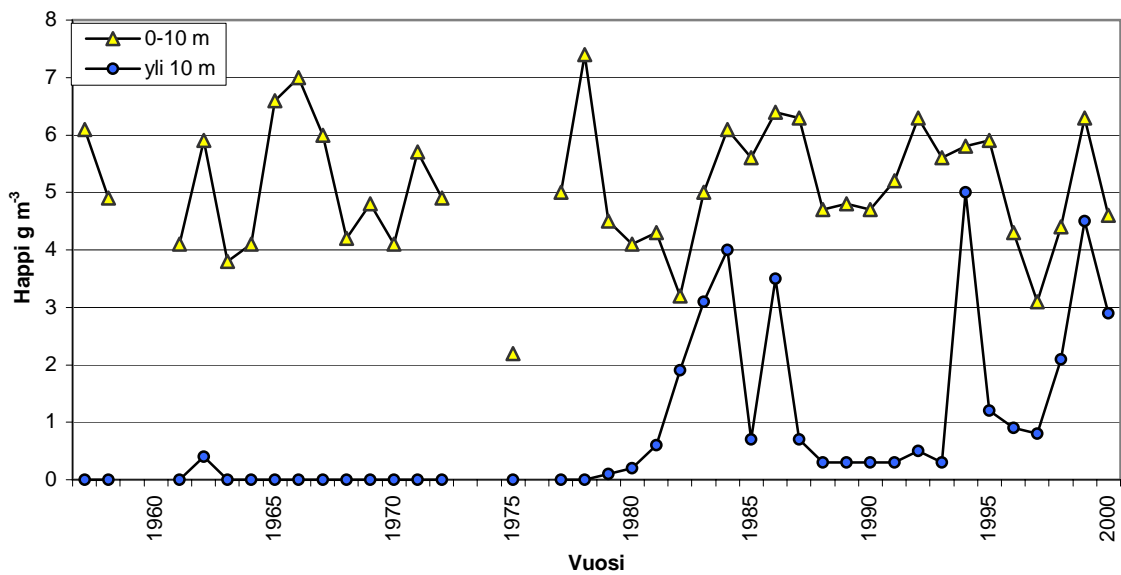
Kuva 17. Päällys- ja alusveden happipitoisuuksien keskiarvot heinä-elokuussa 1957–2000 (lähteet: liite 6).
