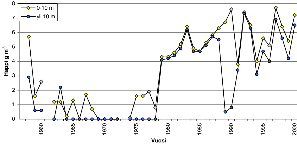
Kuva 16. Pinnan ja pohjan läheisten vesikerrosten happipitoisuuksien keskiarvot maaliskuussa 1958–2000 (lähteet: liite 6).
